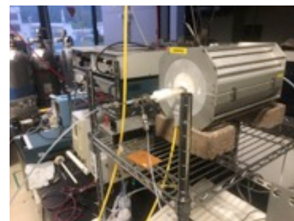
水素分離膜評価装置
