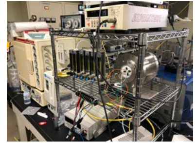
セラミックガスセンサ評価装置
